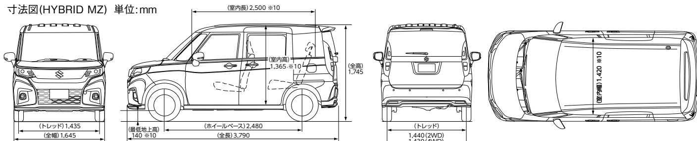
寸法図(HYBRID MZ) 単位:mm
