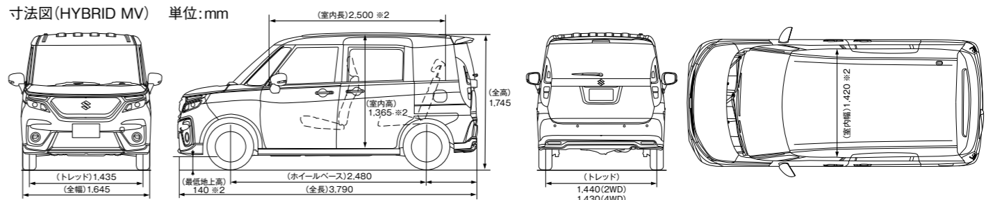
寸法図(HYBRID MV) 単位:mm
