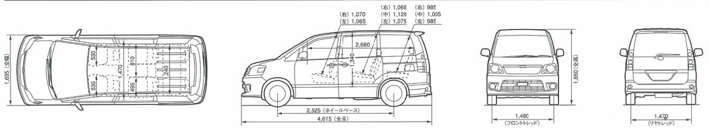
トヨタ ノア S 寸法図 (単位: mm) イラストはS 2WD セカンドシート・マルチ回転シート (シートバックテーブル付・スライド式) です。
