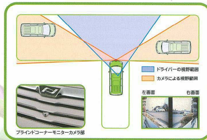
ブラインドコーナーモニターカメラ部
