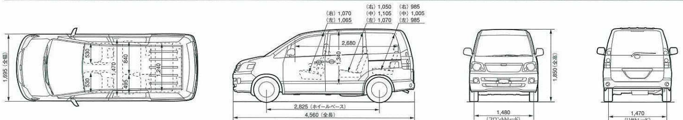
トヨタ ノア S 寸法図 (単位: mm) イラストはS 2WD セカンドシート・マルチ回転シート (シートバックテーブル付・スライド式) です。
