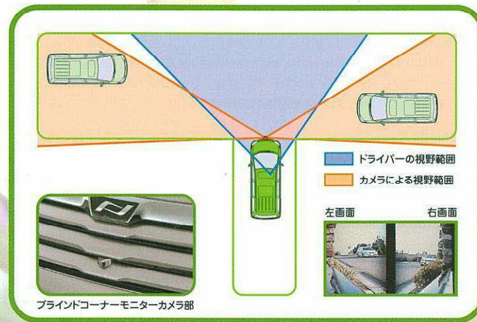
ブラインドコーナーモニター説明図 (イメージ)
