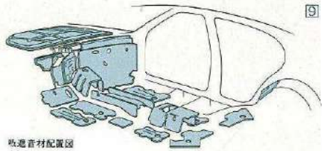
吸音材配置図
