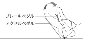
マツダのペダルレイアウト 前輪を前方に移動し、足を自然に伸ばした位置にペダルを配置
