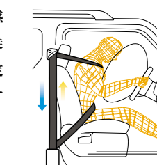
プリテンショナー機構 フォースリミッター機構
