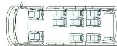
シート配列図(最後列スペースアップシートはね上げ状態)
