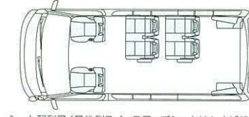
シート配列図 (最後列スペースアップシートははね上げ状態)
