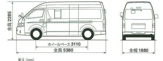
■スーパーロング・ワイドボディ・ハイルーフ
