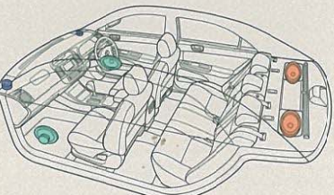
スピーカー配置図
