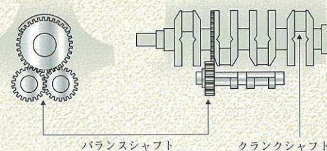
バランスシャフト説明図 5S-FEエンジンに採用のバランスシャフト
