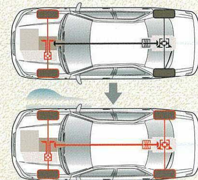
Vフレックスフルタイム4WD説明図 ■駆動輪
