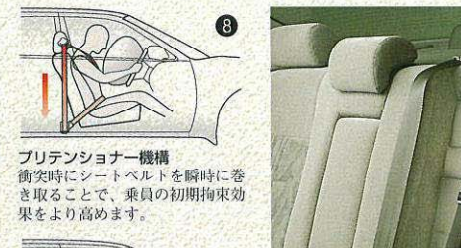
プリテンショナー機構 衝突時にシートベルトを瞬時に巻き取ることで、乗員の初期拘束効果をより高めます。
