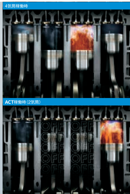
Photo:1.5L TSI® Evoエンジン 写真は機構説明用につき実際のものと一部異なります。
