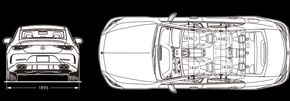
単位: mm
